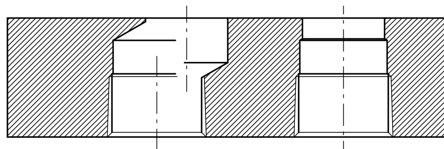
断面A-A'
