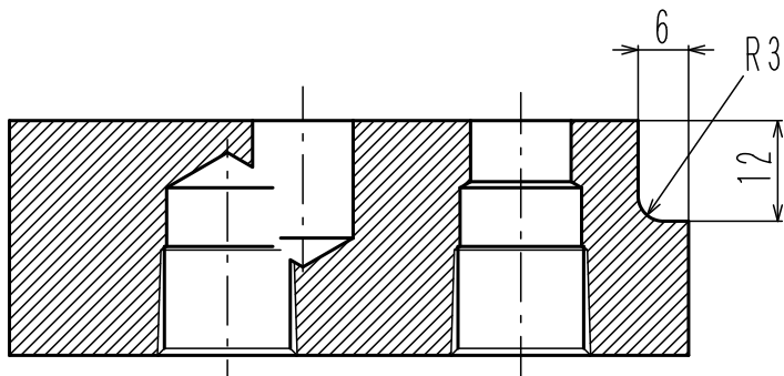
断面A-A'
