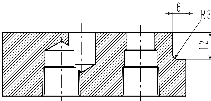
断面A-A'
