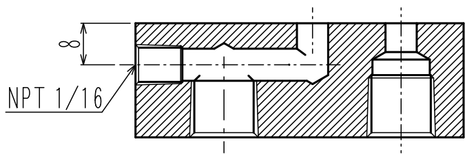
断面 A - A'
