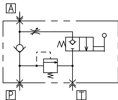
L V M O 回 路 例 (LVMO-303T)
