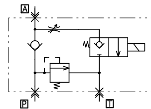
(LVSO-30 ※の回路図)
