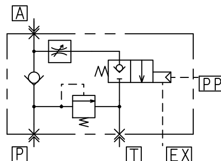
L V P O 回 路 例 (空 圧) (LVPO-303T-AR)
